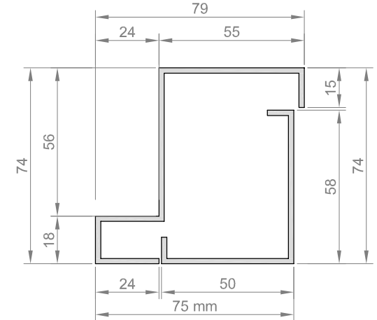
PARTICOLARE TELAIO-CONTROTELAIO RINFORZATO SPESSORE 25/10 - rapp. 1:2
