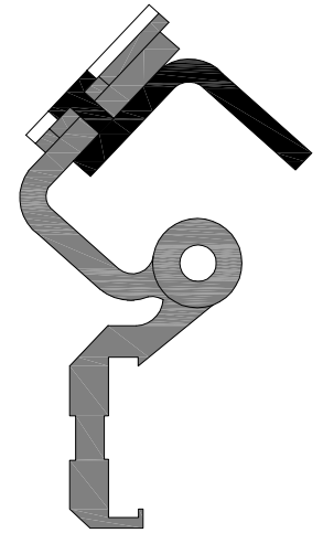
PARTICOLARE CERNIERA A SCOMPARSA - rapp. 1:2
