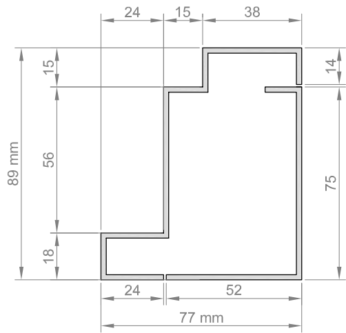
PARTICOLARE TELAIO-CONTROTELAIO - rapp. 1:2
