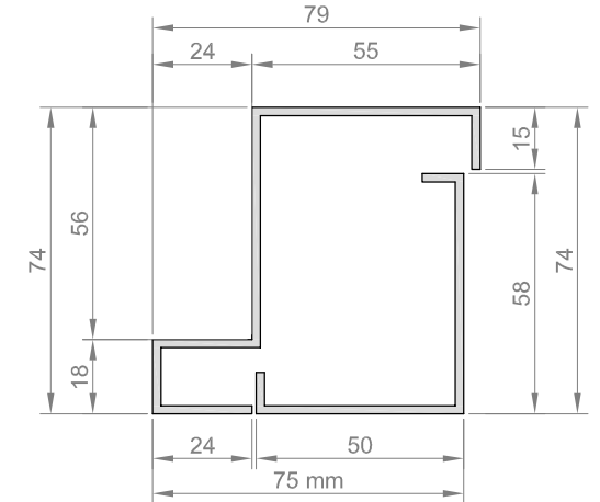
PARTICOLARE TELAIO-CONTROTELAIO - rapp. 1:2
