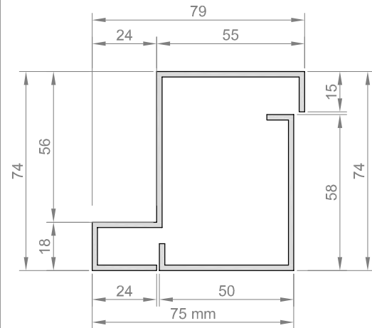
PARTICOLARE TELAIO-CONTROTELAIO - rapp. 1:2
