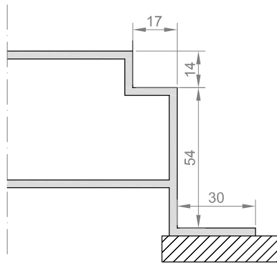
PARTICOLARE BATTUTA CENTRALE - rapp. 1:2
